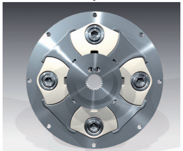
Type 3 / Bauform 3
